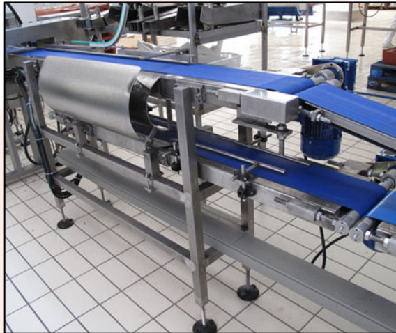
BANDA de LONA CON VOLTEO
