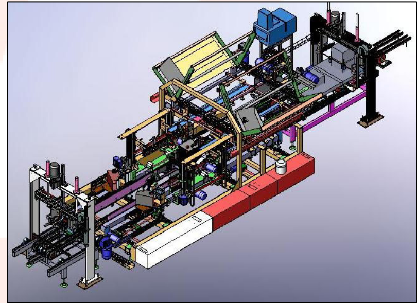
ENCAJADORA AUTOMÁTICA de BALDOSAS CERÁMICAS
