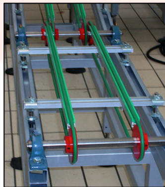
CORREAS TRACCIONADAS POR POLEAS
